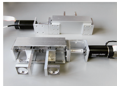
▲バイラテラル・マスタ・スレーブハンド
