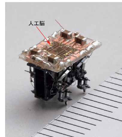
▲ 人工脳を搭載した世界最小の4足歩行ロボット
