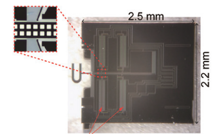
▲ 開発中の静電気力を応用した微細なモータ
