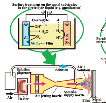
▲ 図1 溶液中で行われる金属表面処理（上）と新しい金属表面処理技術の構想（下）
