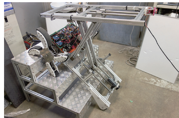
写真1 展開車輪ロボットの階段昇降
