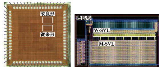
改良形 従来形 改良形 W-SVL M-SVL 低リーク電流を実現するアシスト回路を搭載したSRAMメモリ回路（レイアウト図およびチップ写真）
