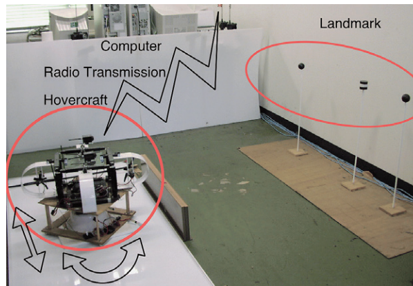
▲ホバークラフト型全方向移動体
