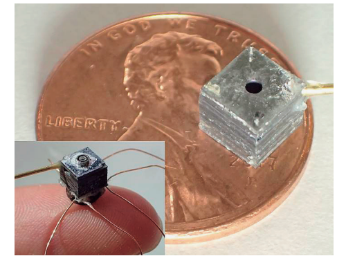
▲ 開発した超小型発電機
