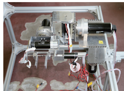
▲6自由度ロボットマニピュレータ
