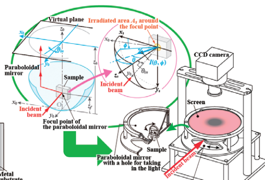
▲ 図2 物体表面の光性質評価装置
