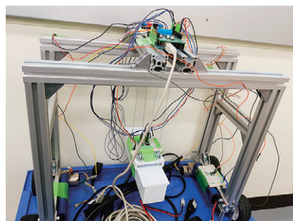
▲ 運搬車両の構造と挙動のシミュレーター
