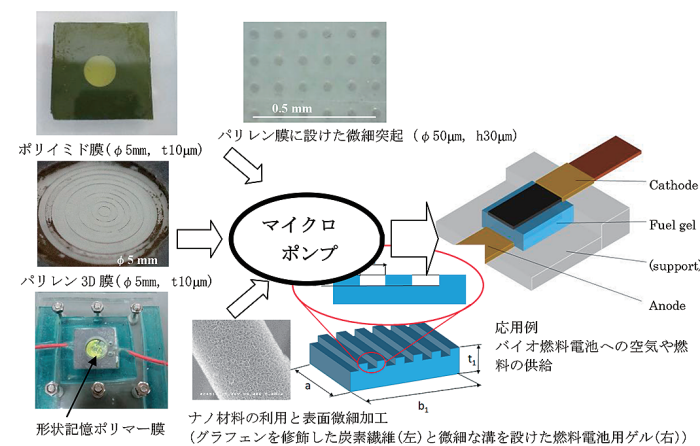
◀ 図1 MEMS 要素技術とマイクロ流体搬送デバイスへの応用。左の膜（ダイアフラム）は液体搬送用、中央上の微細突起は液体を移動させやすくするための表面構造、中央下は表面積を増やすための電極や燃料ゲルの表面構造。右は応用例としてのバイオ燃料電池
