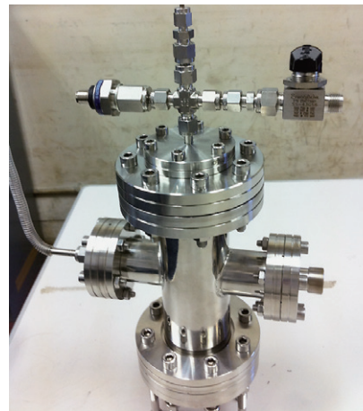
▲ ランキンサイクル用作動流体の熱特性測定装置
