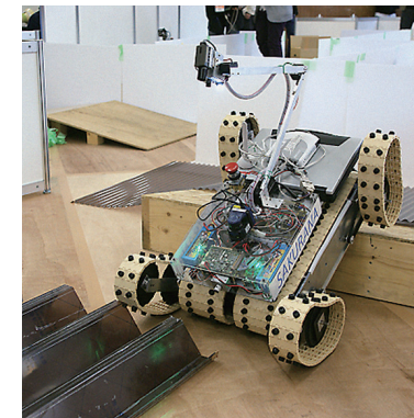
探索型レスキューロボット
